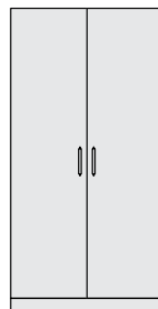
30" Double Robe H: 1800 W: 760 D: 520
